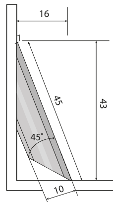
SOCKELLEISTEN KONISCH SWING SKIRTINGS CONICAL SWING
