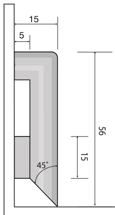
SOCKELLEISTEN KLASSIK SKIRTINGS CLASSIC
